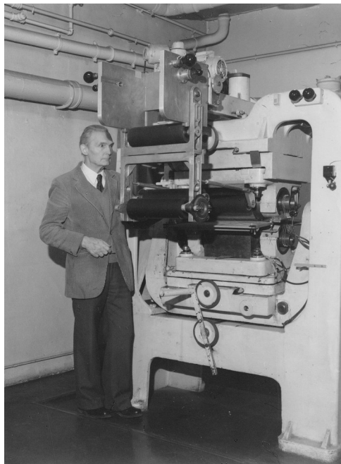
Maurice Bonnet devant la machine à gaufrer, calendeuse pour « film gaufré » qui a donné son nom au laboratoire de l'inventeur à son arrivée au CNRS en 1961.
