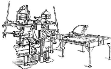
Рис. 202. Стереопланграф
