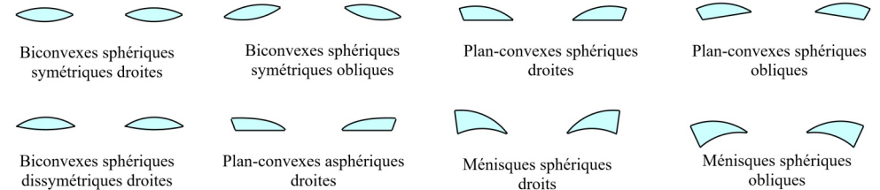
Fig. 3 - Exemples de type de lentilles
