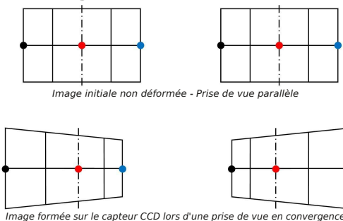
Fig. 1 : Déformations engendrées par la prise de vue en convergence
