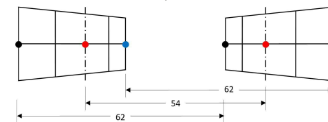
Fig. 2 : Modifications de la distance des points homologues par la prise de vue en convergence Au centre de l'image la distance entre homologues est plus faible que sur les bords
