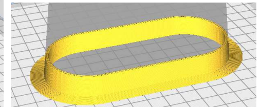
Technique de la bordure : monocouche périphérique de matériau, solidaire de la pièce.
