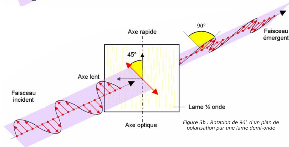
Figure 3a : Rotation d'un plan de polarisation par une lame demi-onde sous un angle quelconque
