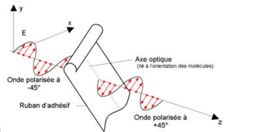
Figure 6c : Si l'adhésif est orienté à 135° par rapport au plan de polarisation, il sera retourné de 180°, donc sans effet apparent.
