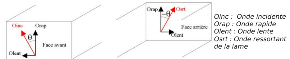
Figure 2 : Représentation vectorielle des ondes entrant et sortant d'une lame demi-onde
