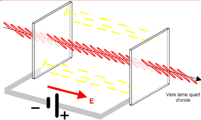
Figure 3 : Ligne paire. En présence d'un champ électrique E, les molécules de cristaux liquides s'alignent dans la direction de ce champ, la structure en hélice est détruite, aucune rotation de polarisation ne se produit.
