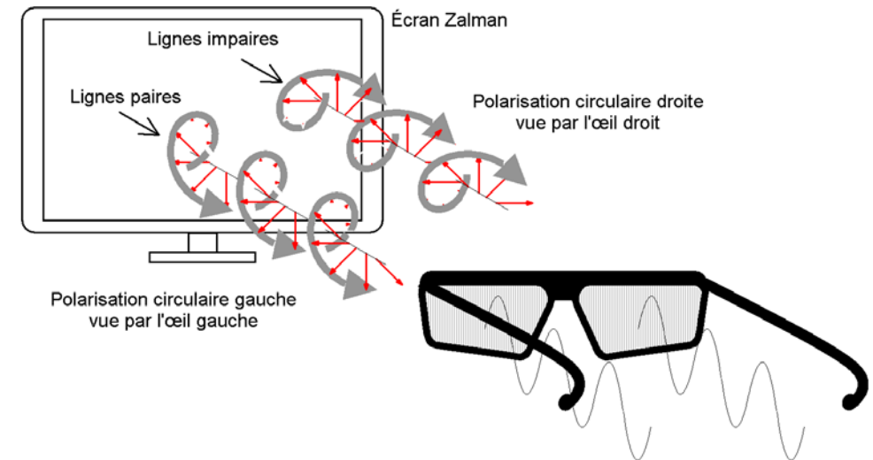
Figure 4 : La lumière émise par l'écran Zalman est polarisée circulairement. Le sens de rotation permet de distinguer les images droite et gauche.
