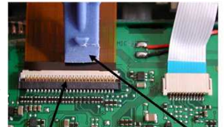
Connecteur écran LCD : utiliser un outil adapté pour soulever l'agrafe de verrouillage de la nappe
